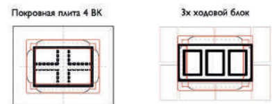
Варианты установки дефлектора 39/53 на типовые комбинации вентканалов
