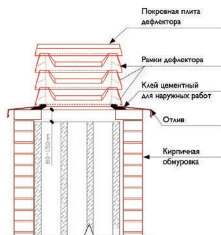
Варианты установки дефлектора 39/53 на типовые комбинации вентканалов
